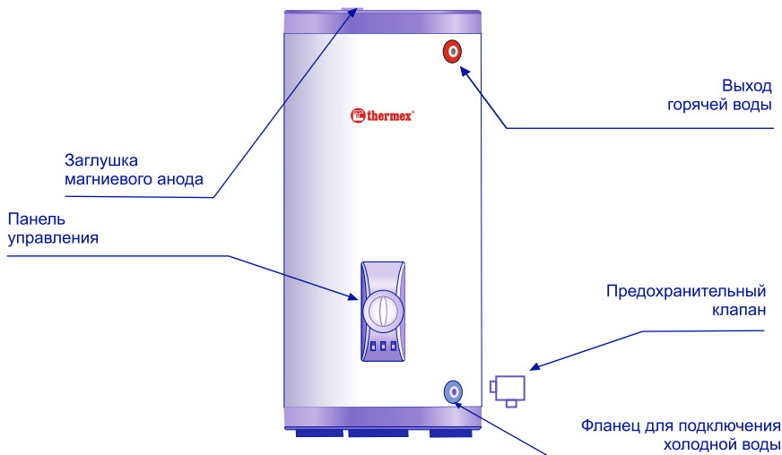
Рис. 1. Схема подключений
